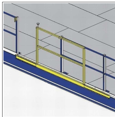
Schiebegeländer
