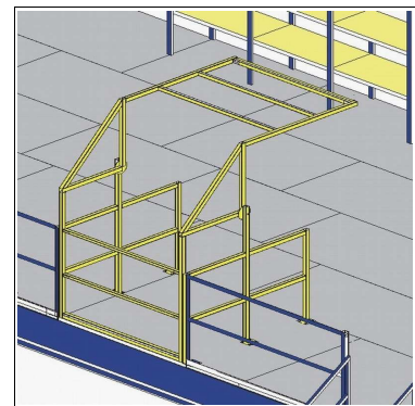
Schwenkschleuse
